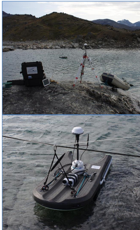
Imeqarfii avataanit kuuffiqineqarlutik immerneqarnerinik uuttortaanerit atorlugit GSs-iligaasumik uuttortaasiaq nutaajusoq ADCP, atorlugu sukkuinerusumik pitsaane-rusumillu uuttortaasinnaaneq periarfissaalerpoq.
