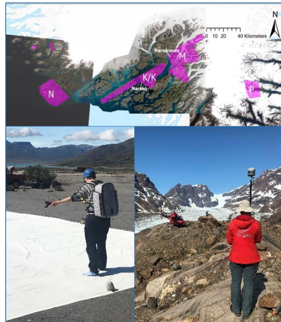
Silaannakkut angalasinnaanermut attuumassuteqartunik nu-natta Kujataani suliaqarnermi nunamiit aqutsinermi toqqa-mavissanik pilersitsineq.
